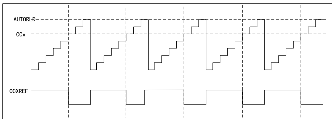
图 42 PWM1 向上计数模式的时序图
