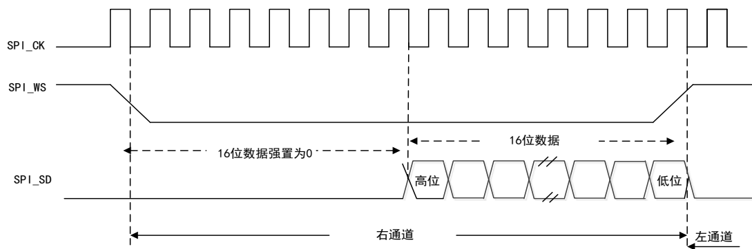
图 100 LSB 对齐标准下（16 位扩展至 32 位）
