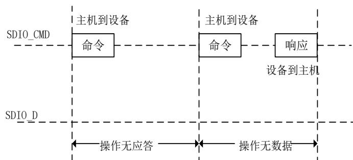
图 114 SDIO（多）数据块读操作
