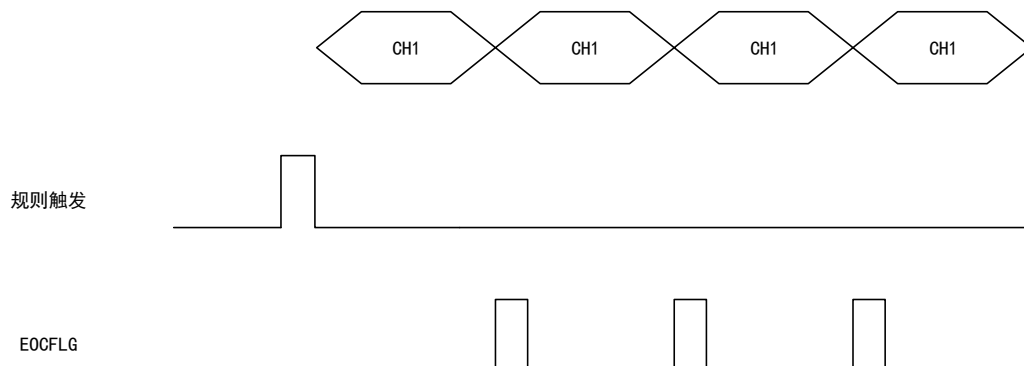
图 121 连续转换模式时序图
