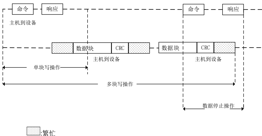
图 115 SDIO（多）数据块写操作
