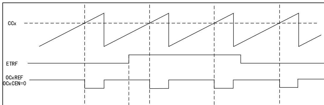
图 36 OCxREF 时序图
