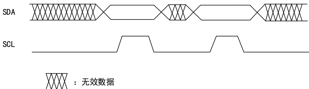
图 84 SDA 时序图
