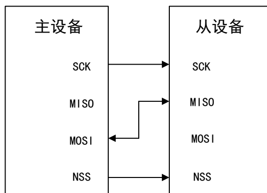
图 91 双向线连接
