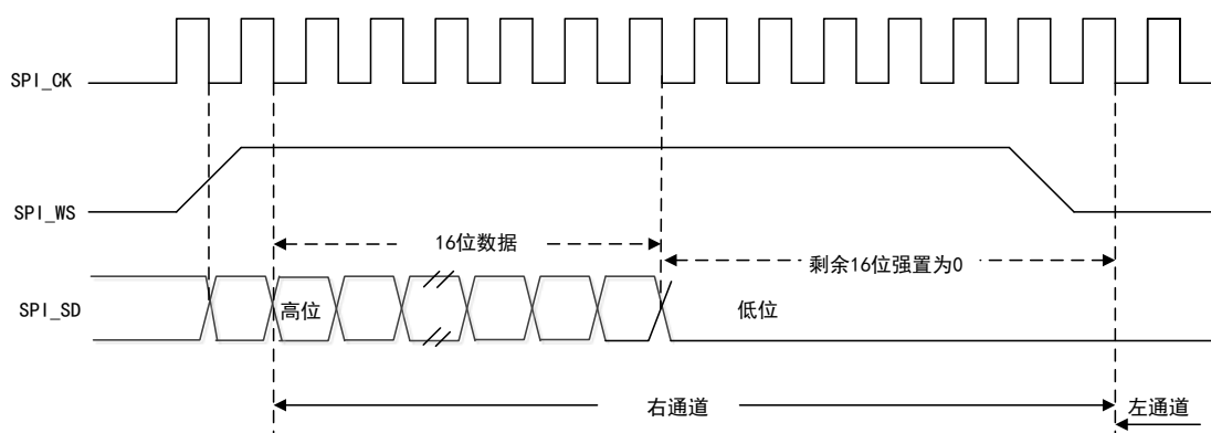
图 94 I2S 飞利浦协议波形（16 位扩展至 32 位）
