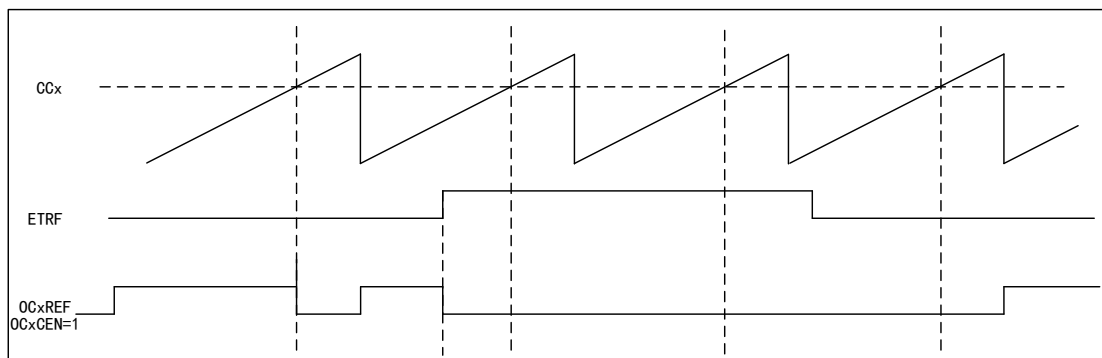
图 53 OCxREF 时序图
