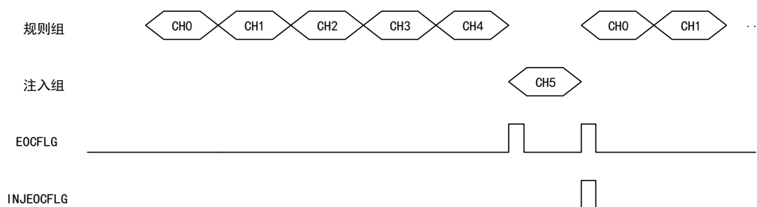
图 125 自动注入时序图
