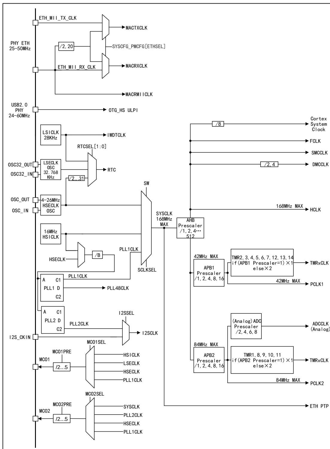
图 6 APM32F405/415xG、APM32F407/417xExG 时钟树
