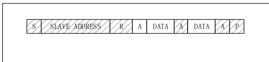
图 83 主机由从机读取数据
