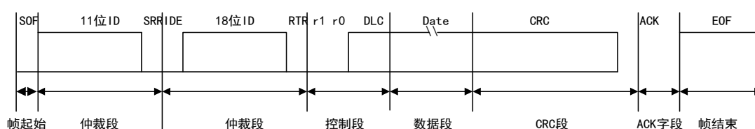
图 104 扩展数据帧
