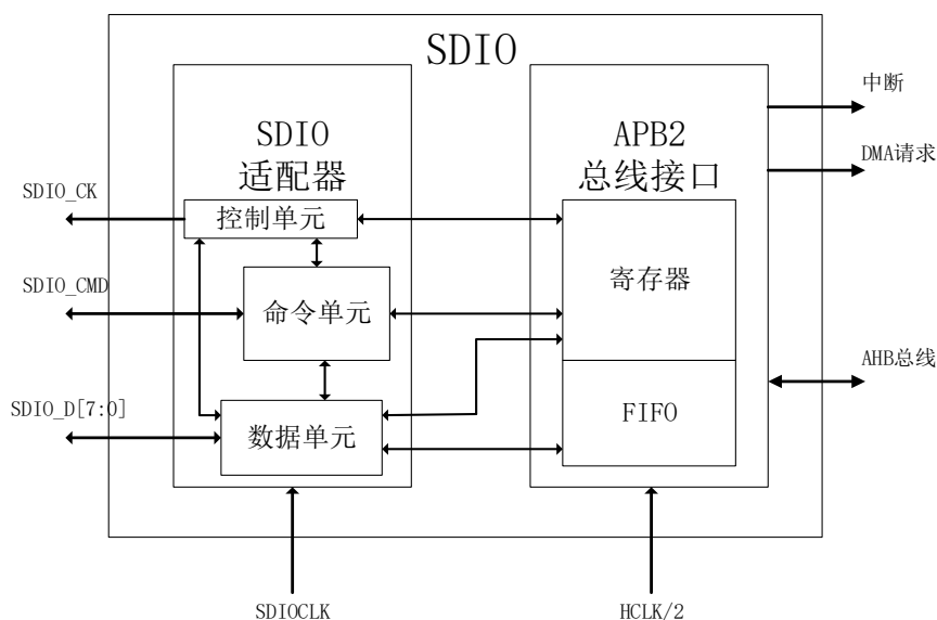
图 112 SDIO 结构框图如图
