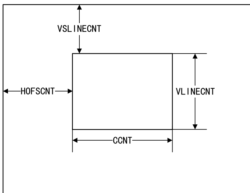
图 68 裁剪窗口时的参数定义
